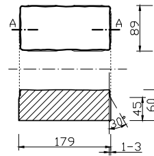
PRZEKRÓJ A-A
