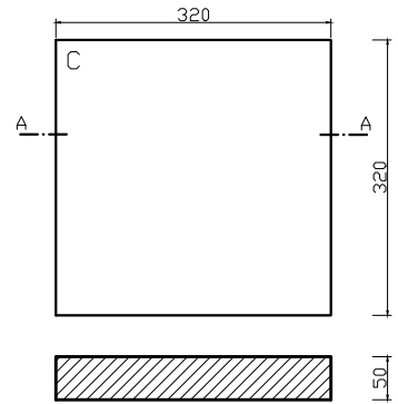
PRZEKRÓJ A-A
