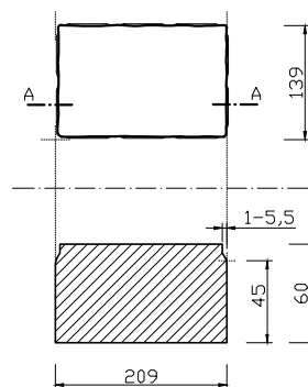
PRZEKRÓJ A-A
