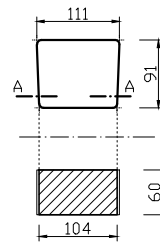
PRZEKRÓJ A-A
