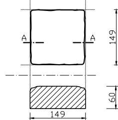
PRZEKRÓJ A-A
