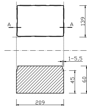
PRZEKRÓJ A-A
