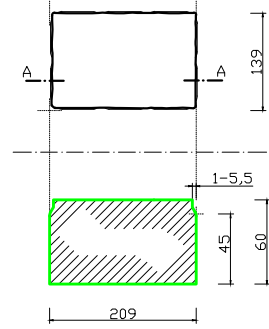
PRZEKRÓJ A-A
